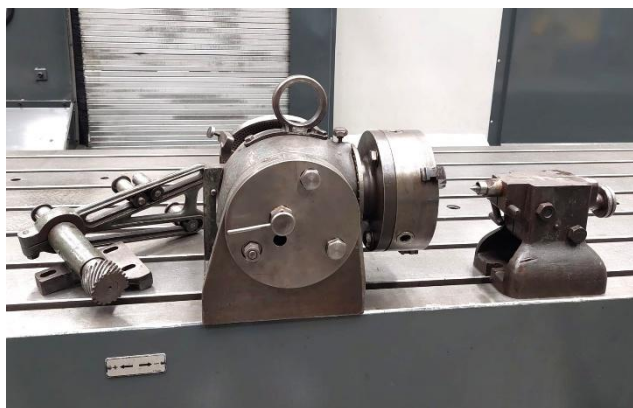
Ref. 280/V222 Divisor con plato de torno universal 3 garras Ø 190 mm. Puede trabajar en horizontal y vertical. Equipado con punto y guitarra. Precio: 1.000 €
