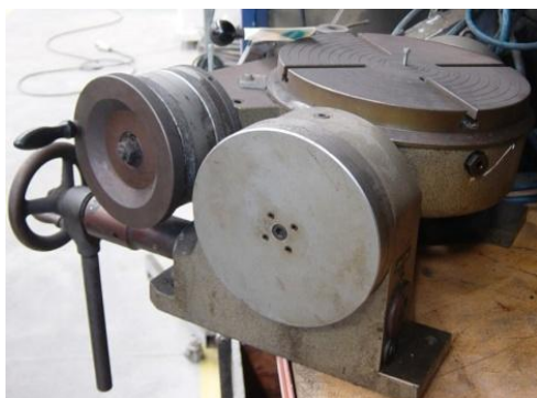
Ref. 280/V026 Plato divisor basculante L.HAUS AG Ø 250 mm Precio 900 €
