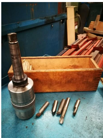
Ref. 280/V187 Cabezal de mandrinado D-100 Cono Morse-2 Precio 100 €
